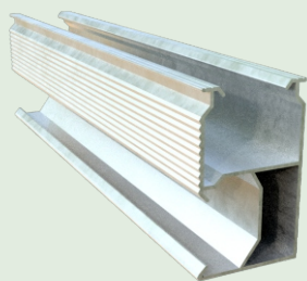
PERFIL C COD.: IZI003 Material: Alumínio T5 - 6060
