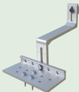
GANCHO P/ TELHA CERÂMICA COM SUPORTE CÓD.: IZI301
