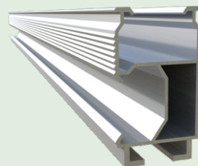
PERFIL REFORÇADO Cod.: IZI009 Material: Alumínio T5 - 6060
