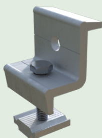
GRAMPO TERMINAL Cod.: IZI201 30mm a 40mm Material: Alumínio T5 - 6060 Parafuso Inox 304 A2
