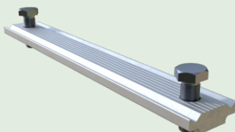
JUNÇÃO DE PERFIL Cod.: IZI211 Material: Alumínio T5 - 6060 Parafuso Inox 304 A2
