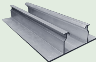
PERFIL BASE RETA COD.: IZI008 Material: Alumínio T5 - 6060
