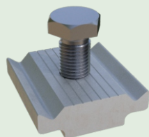
PARAFUSO INOX COD.: IZI210 Parafuso e Arruela Inox 304 A2 Porca Alumínio T5 - 6060
