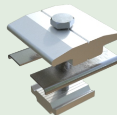
GRAMPO INTERMEDIÁRIO Cod.: IZI-200 Material: Alumínio T5 - 6060 Parafuso Inox 304 A2
